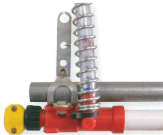
엔드키트 / 자동개폐
