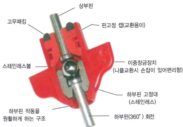
〈 니플 단면 상세도 〉
