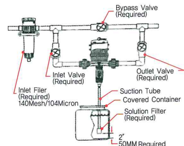
〈 설치방법 예제그림 〉
