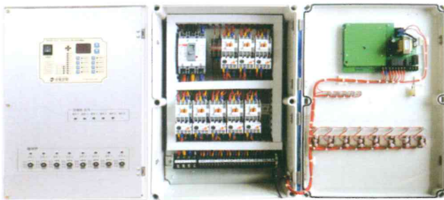
대형헨 콘트롤(5단계)
